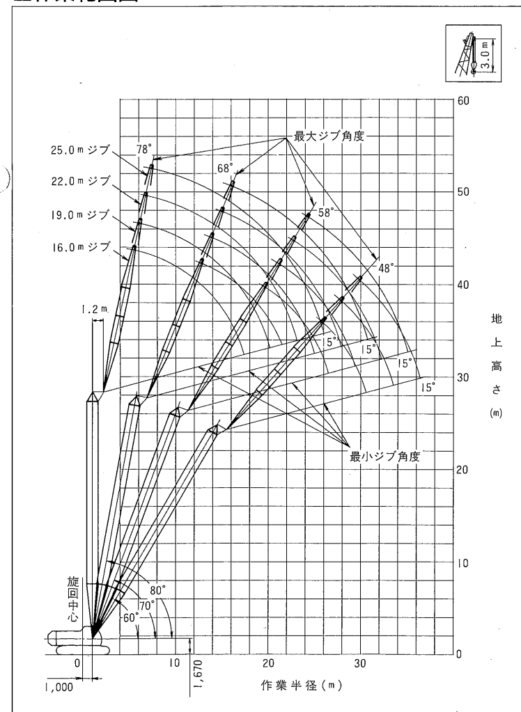
■作業範囲図
