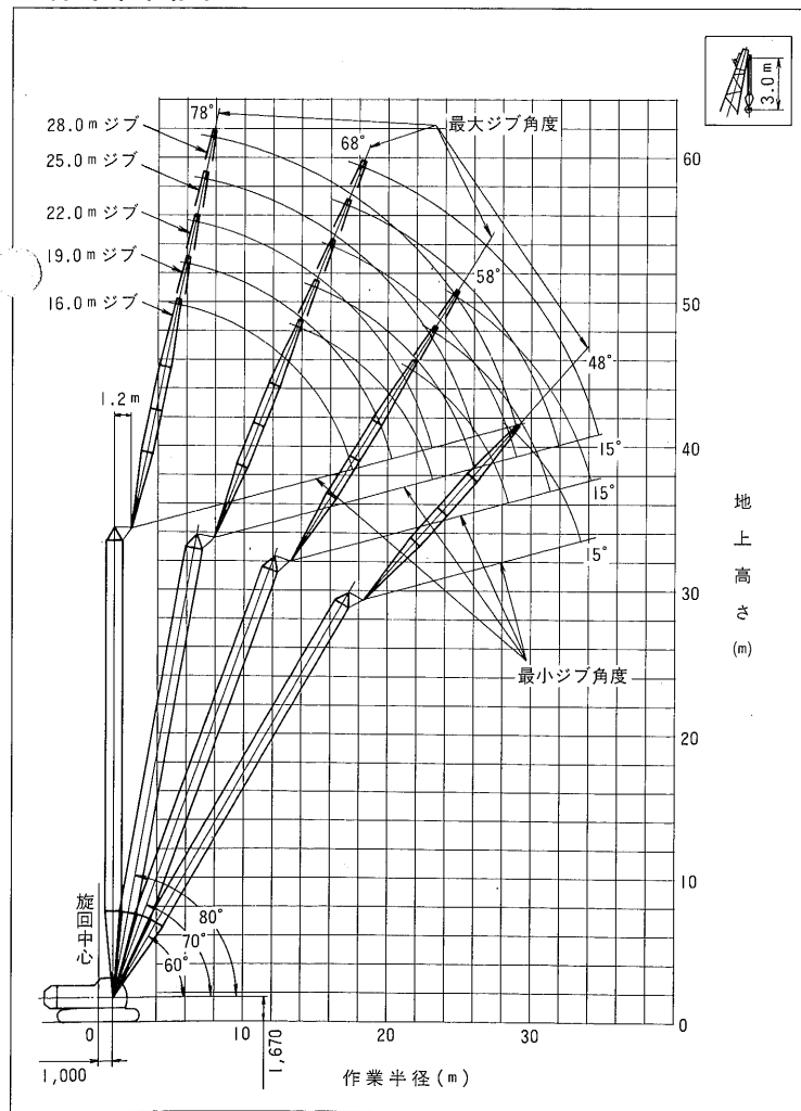
■作業範囲図
