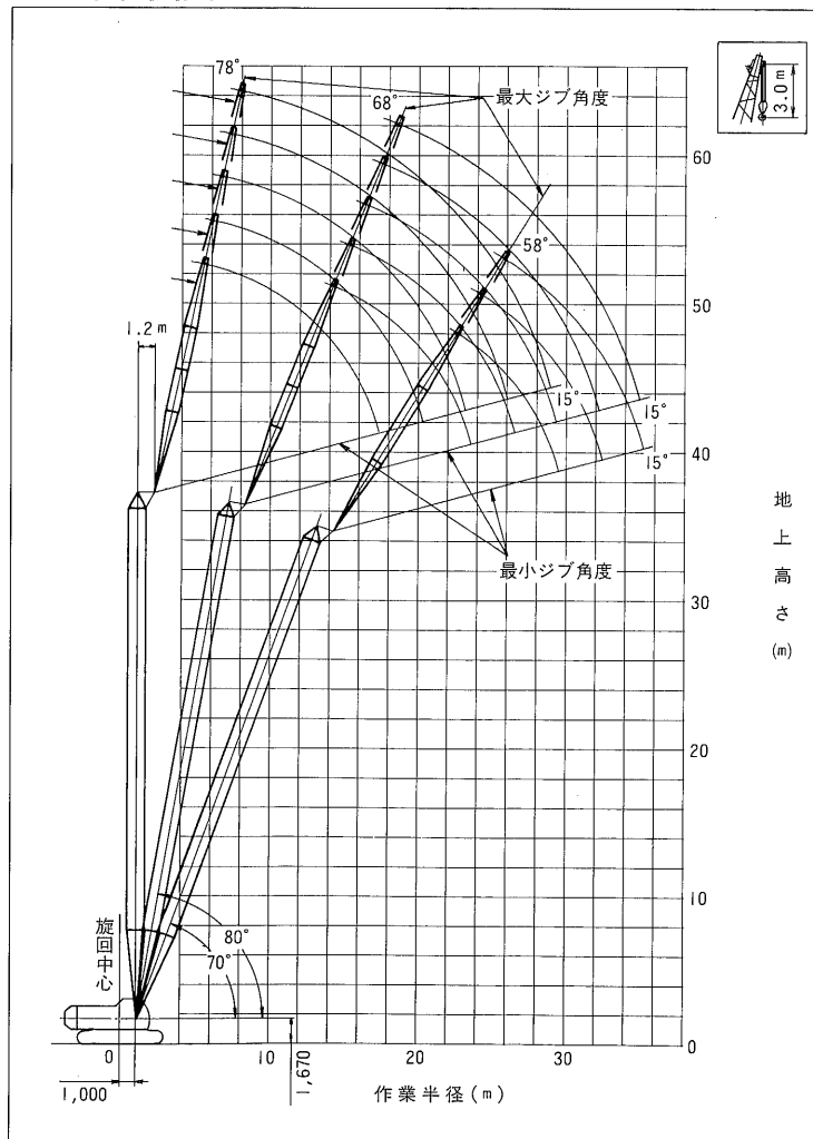
■作業範囲図
